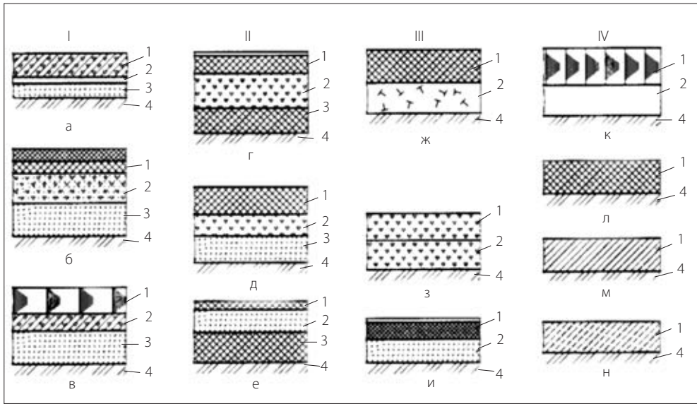
Рисунок 5.12. Конструктивные слои одежд для автомобильных дорог I (а–в), II (г–е), III (ж–и), IV (к–н) категорий: а — цементобетонные монолитные и сборные; б — асфальтобетонные из горячих и теплых смесей; в — мостовые из брусчатки, мозаики на каменном или бетонном основании; г — щебеночные из прочных щебеночных материалов подобранного состава с минеральным порошком или без него, обработанные в смесителе вязкими органическими вяжущими; д — щебеночные (гравийные), обработанные по способу пропитки; е — из холодного асфальтобетона; ж — из грунтов, обработанных в установке вязким битумом; з — щебеночные (гравийные), шлаковые; и — грунтовые и из местных слабых материалов, обработанных органическими вяжущими; к — мостовые из булыжного или колотого камня; л — грунтовые, укрепленные местными скелетными материалами (гравием, щебнем и др.); м — грунтовые подобранного гранулометрического состава; н — грунтовые неукрепленные; 1 — дорожное покрытие; 2 — основание; 3 — дополнительный слой основания; 4 — грунтовое основание
