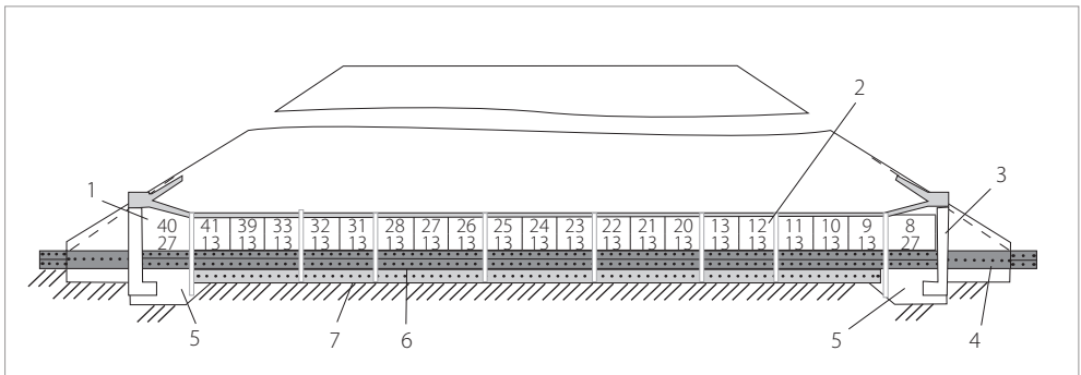
Рисунок 5.14. Водопропускная труба: 1 — коническое звено трубы; 2 — звенья; 3 — порталный блок оголовка; 4 — лоток из монолитного бетона; 5 — песчано-гравийная подготовка; 6 — щебеночная подготовка; 7 — блоки фундамента
