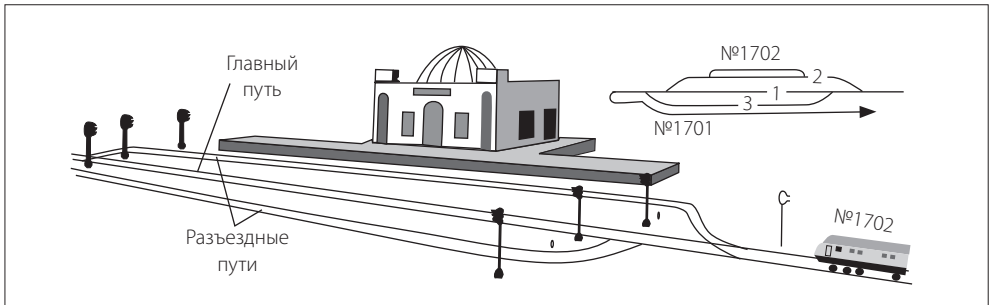
Рисунок 2.17. Разъезд поперечного типа в путях
